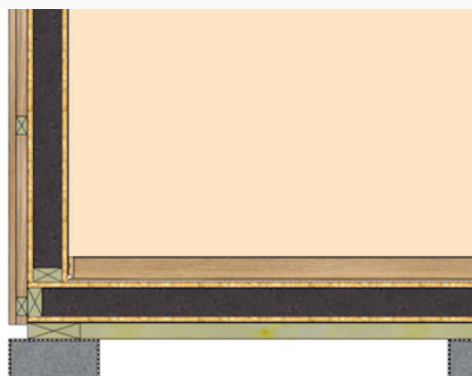
Ściana zewnętrzna i strop zerowy
